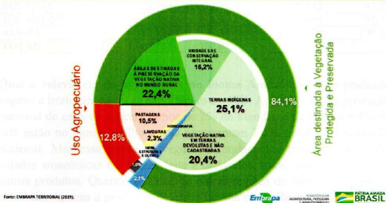
Figura 1. Áreas de vegetação nativa, áreas exploradas, água e outros no bioma Amazônia.
